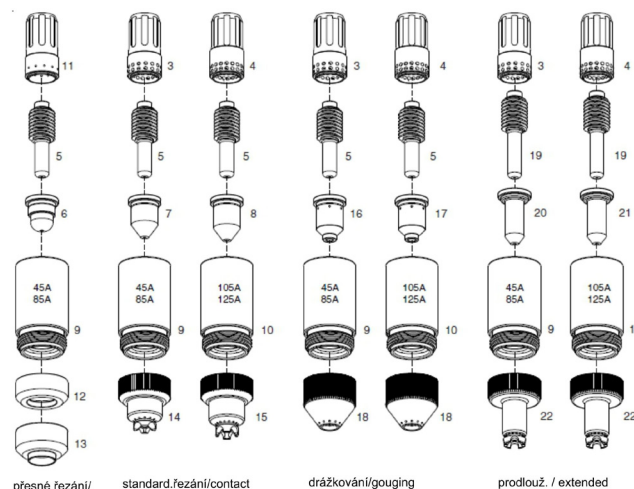
přesné řezání/precision Cut standard.řezání/contact drážkování/gouging prodlouž. / extended
